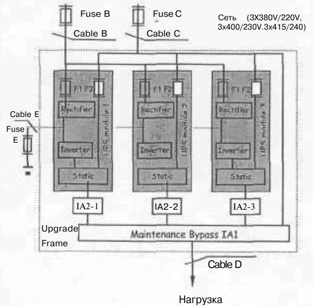
Версия по требованию (Двойной входной кабель)
