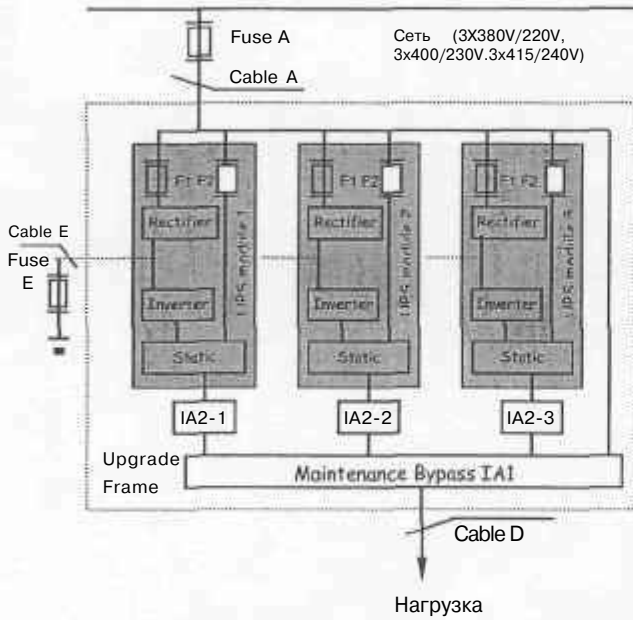
Стандартная версия (Одиночный входной кабель)
